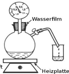
Abb. 2 (rechts). Verdrängung der Luft aus dem Dampfdruckmessgerät.
