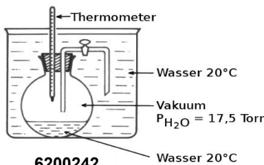
Abb. 6 (rechts). Nachweis der Kondensationswärme von Wasser
