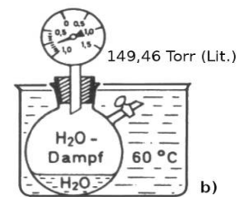
Abb. 7. Messung des Dampfdruckes von Wasser bei 50°C (a) und bei 60°C (b) zur Berechnung der Verdampfungswärme.
