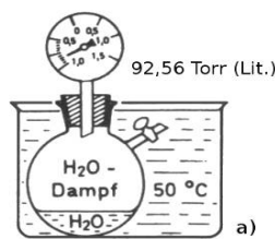
Abb. 7. Messung des Dampfdruckes von Wasser bei 50°C (a) und bei 60°C (b) zur Berechnung der Verdampfungswärme.
